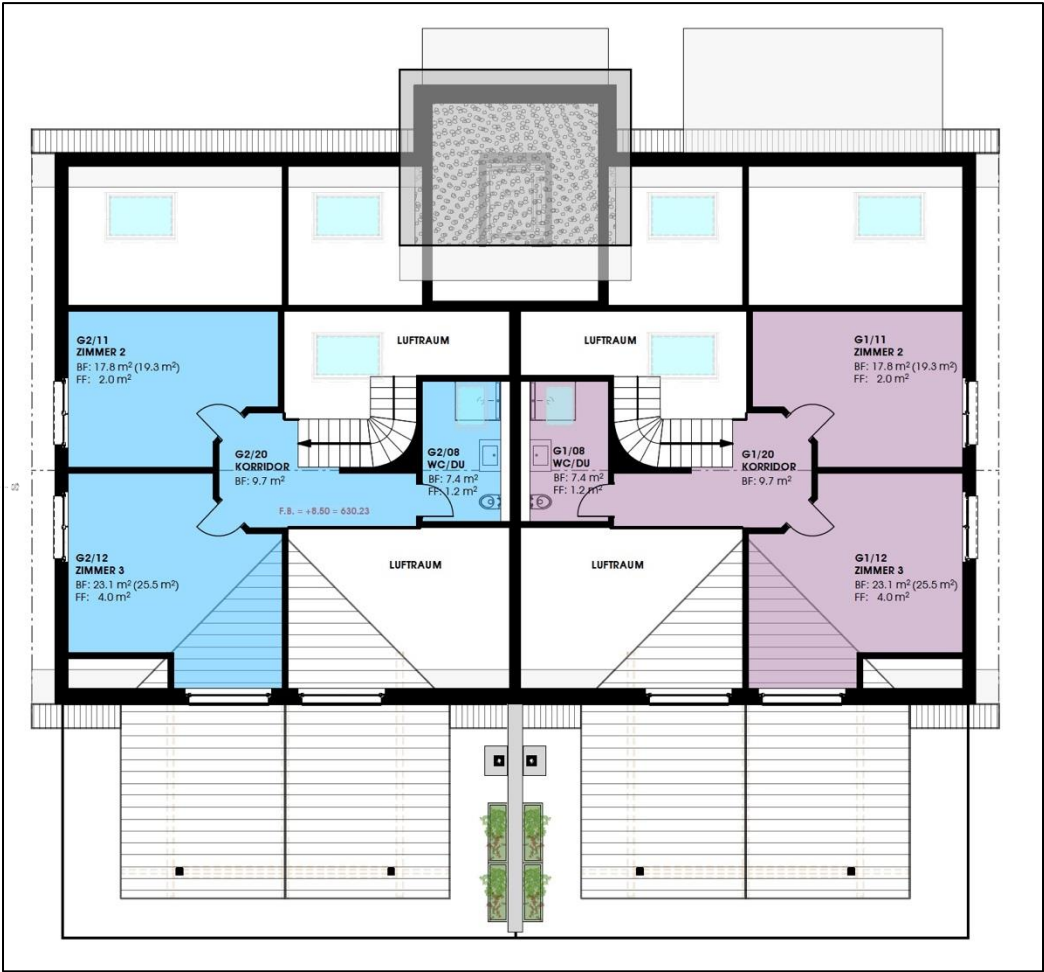
Galeriegesschoss E5 & E6
