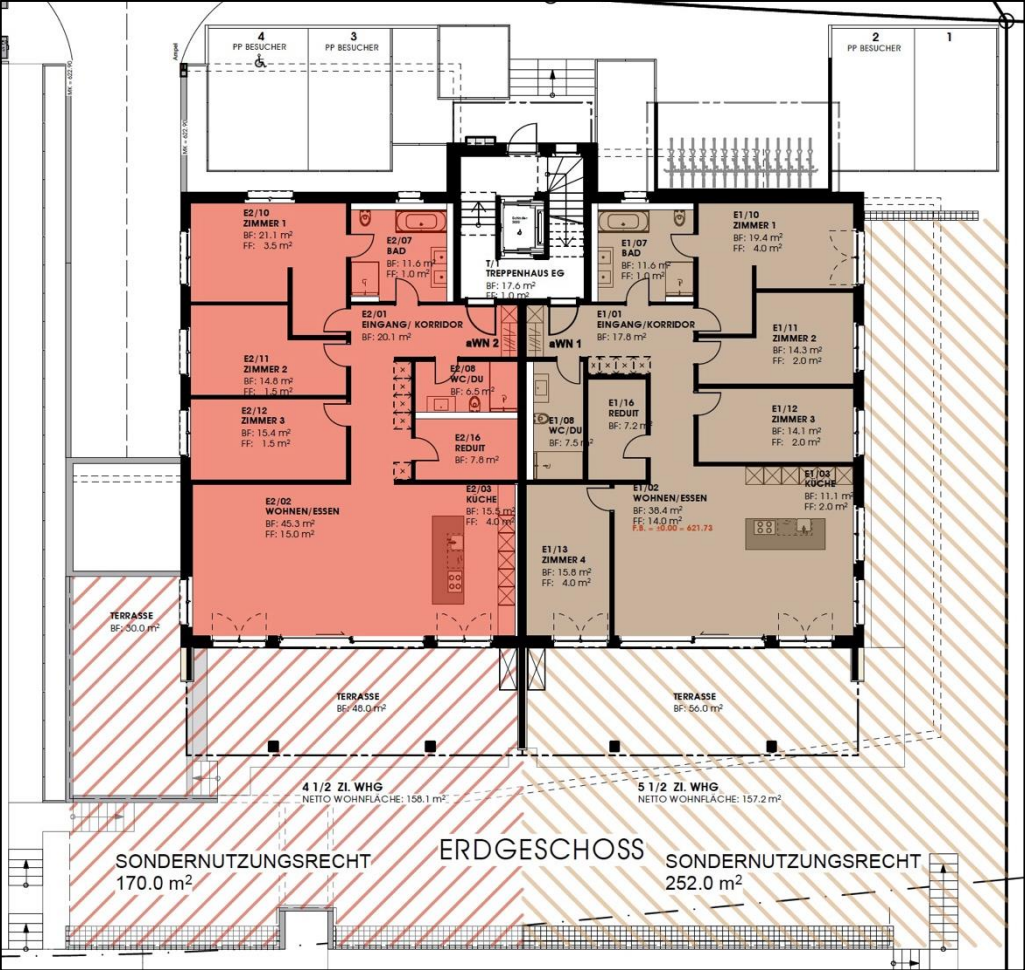
Erdgeschoss E2 (kupfer) & E1 (braun)
